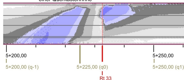
Abbildung 2: Wasserfilmdicken in einem Verwindungsbereich mit Anordnung einer Querkastenrinne
